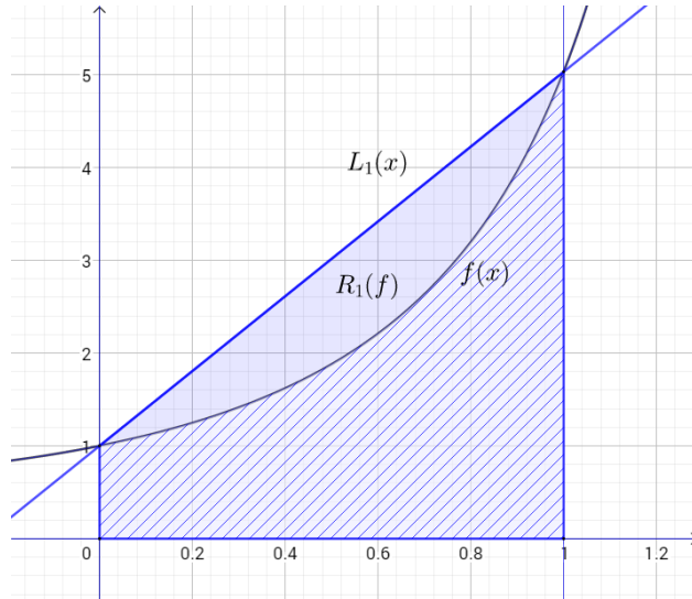
Слика 6.1: Апроксимација интеграла функције \frac{e^x}{\cos x} на интервалу [0, 1] основном трапезном формулом
