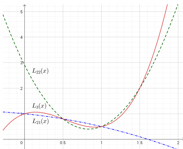
Слика 4.4: Лагранжови интерполациони полиноми
