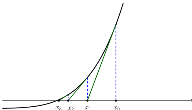
Слика 2.3: Геометријска интерпретација Њутнове методе
