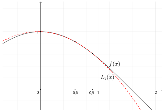
Слика 4.2: Интерполациони полином L_2(x) и функција f(x) = \cos x
