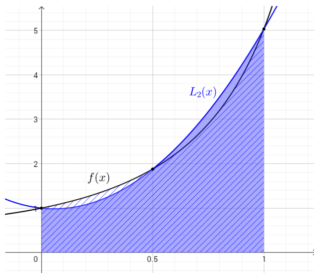
Слика 6.2: Апроксимација интеграла функције \frac{e^x}{\cos x} на интервалу [0, 1] основном Симпсоновом формулом
