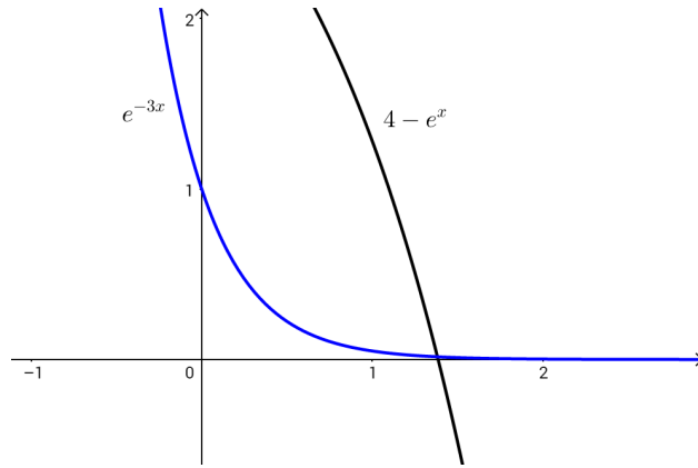
Слика 2.4: Локализација позитивног решења једначине e^x + e^{-3x} - 4 = 0
