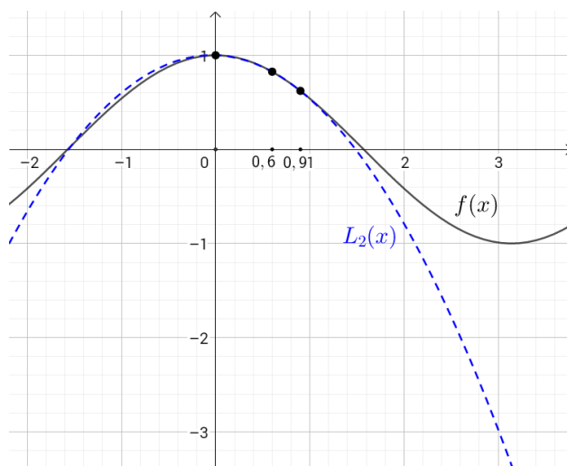
Слика 4.6: Екстраполација функције \cos x
