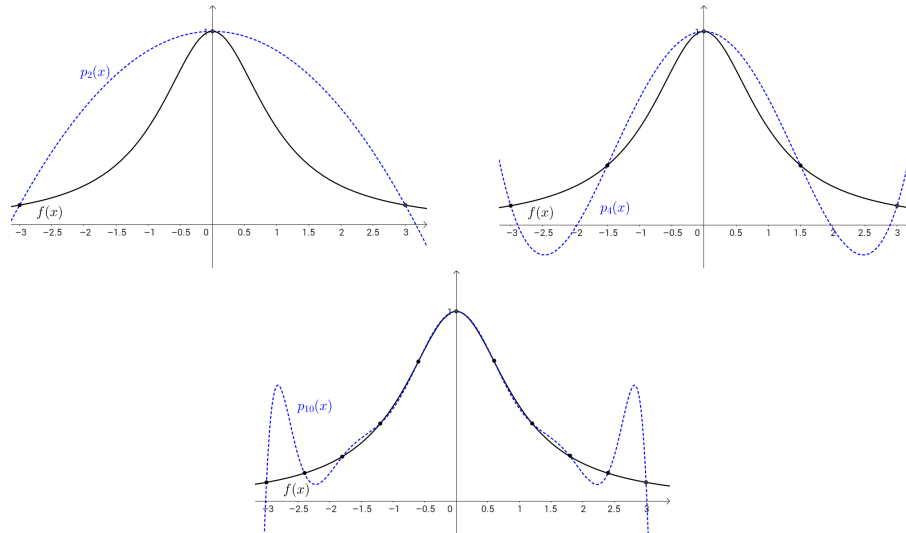
Слика 4.5: Интерполациони полиноми p_2, p_4, p_{10} за функцију f(x) = \frac{1}{1+x^2}
