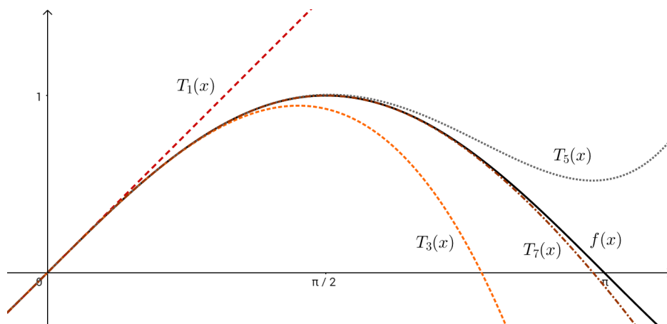
Слика 1.1: Апроксимације функције \sin(x) Тејлоровим полиномима
