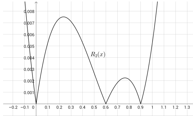
Слика 4.3: Оцена грешке интерполације R_2(x) .
