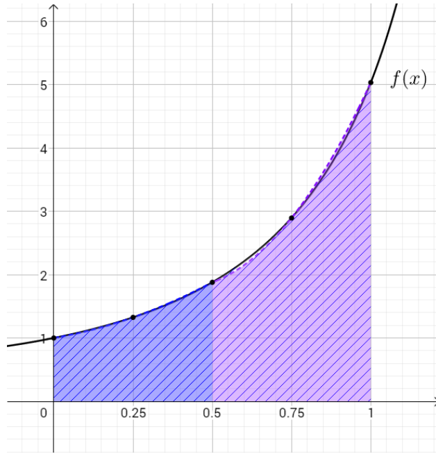
Слика 6.4: Апроксимација интеграла функције \frac{e^x}{\cos x} на интервалу [0, 1] Симпсоновом формулом
