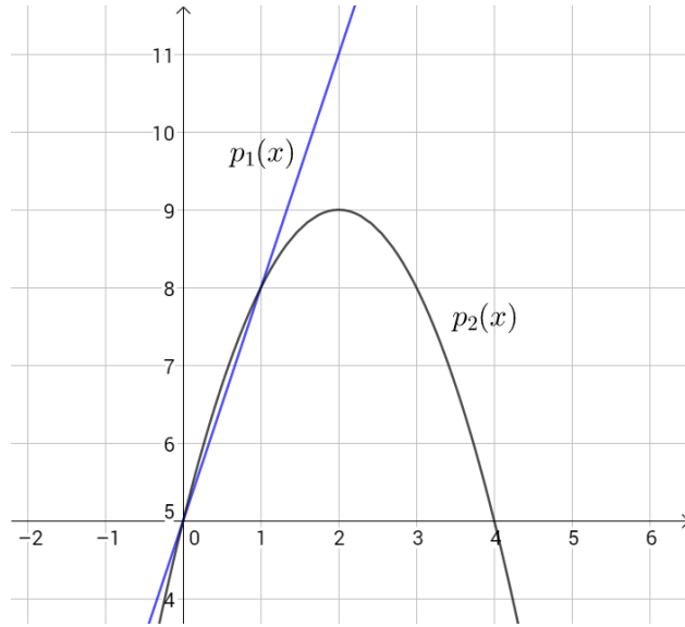
Слика 4.1: Интерполациони полиноми p_1 и p_2 , пример 2
