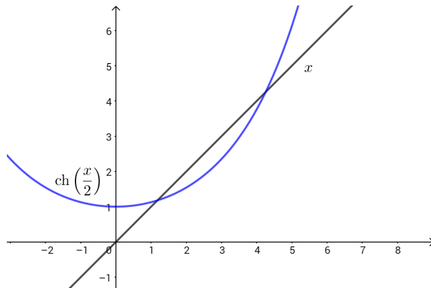
Слика 2.2: Локализација решења једначине \operatorname{ch}\left(\frac{x}{2}\right) - x = 0
