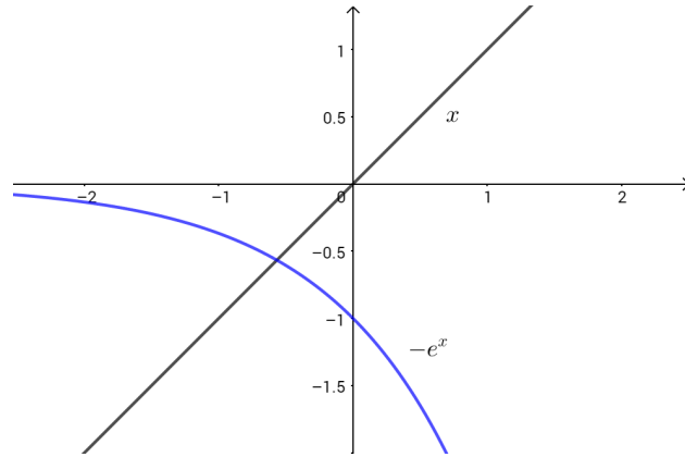
Слика 2.5: Локализација решења једначине x + e^x = 0
