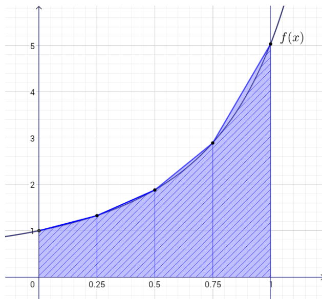
Слика 6.3: Апроксимација интеграла функције \frac{e^x}{\cos x} на интервалу [0, 1] трапезном формулом
