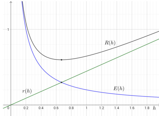
Слика 5.1: Грешке за формулу диференцирања унапред
