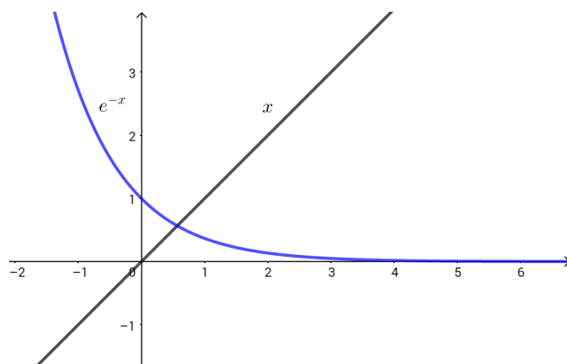
Слика 2.1: Локализација решења једначине e^{-x} - x = 0
