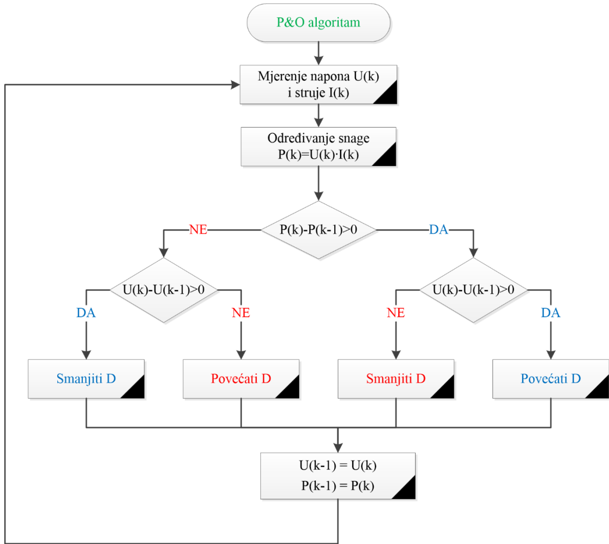
Slika 9. Dijagram toka P&O MPPT algoritma
