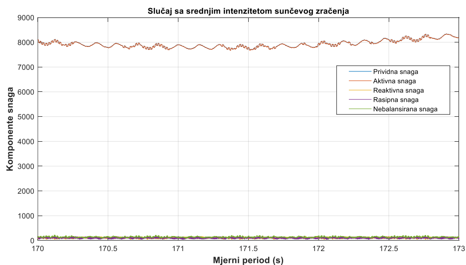
Slika 59. Izračunate komponente snaga pri srednjem intenzitetu sunčevog zračenja
