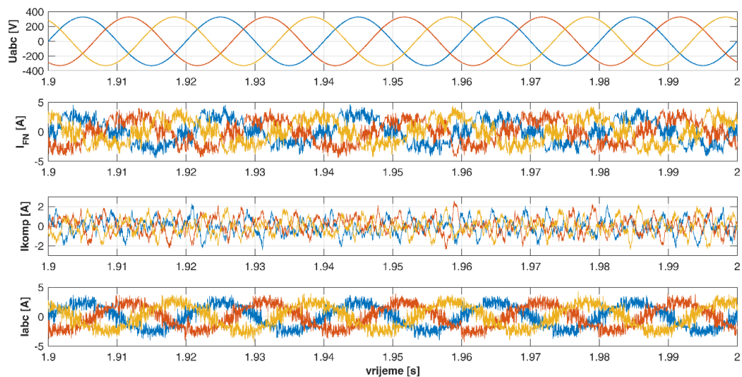
Slika 67. Talasni oblici mrežnog napona i struja FN invertora, kompenzatora i mreže pri slabo opterećenom FN invertoru
