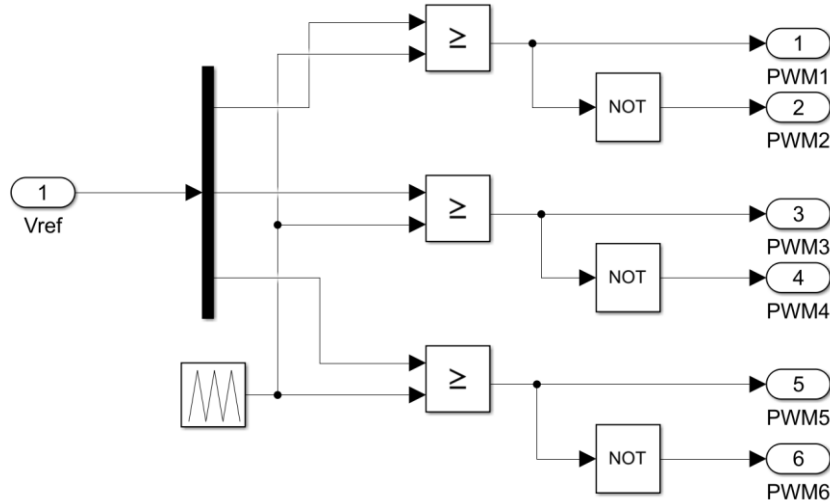
Slika 13. Model trofazne sinusne širinsko-impulsne modulacije
