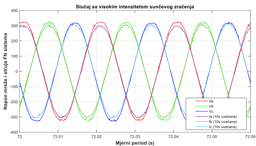
Slika 53. Talasni oblici izmjerene mrežne napona i injektirane struje FN sistema za slučaj sa visokim intenzitetom sunčevog zračenja
