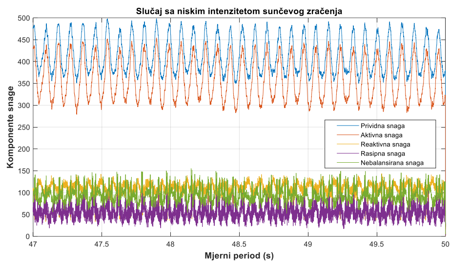
Slika 57. Izračunate komponente snaga pri niskom intenzitetu sunčevog zračenja
