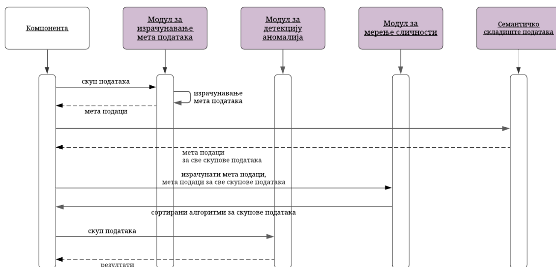
Слика 15: Дијаграм секвенци рада компоненте у фази закључивања. Процес се састоји од израчунавања мета података, рачунања удаљености између скупова података коришћењем мета података и затим одлучивања. Након тога се скуп података евалуира одабраним алгоритмом и врши се валидација добијених резултата.
