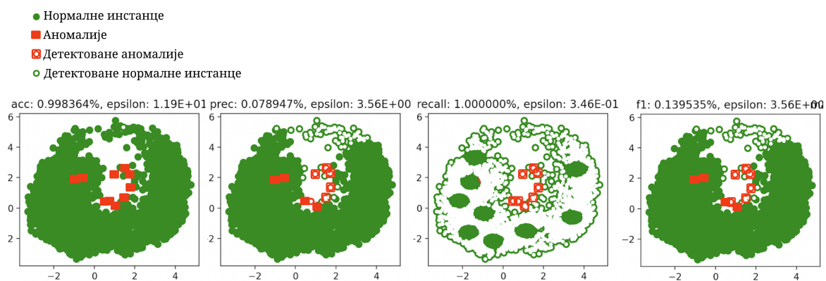
Слика 22: Кластеризација методом К-средњих вредности за различите оптимизационе метрике над једним скупом података. Показано је да одређене оптимизационе метрике иако имају добре перформансе не детектују аномалије у подацима или детектују нормалне инстанце као аномалије.
