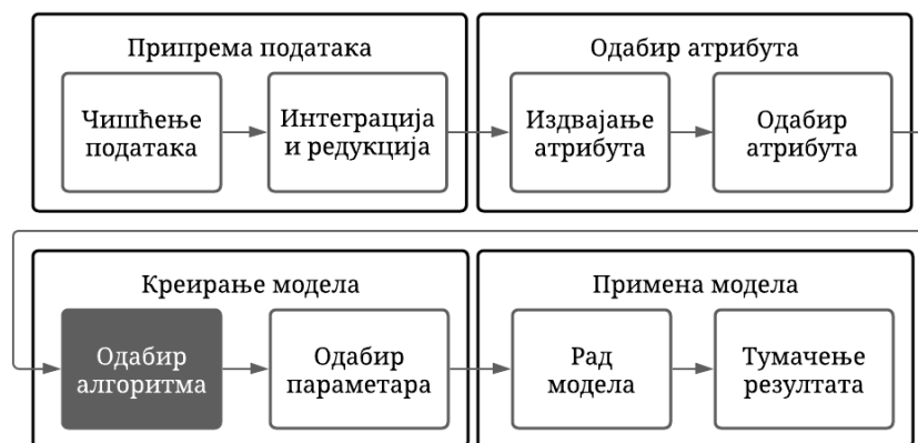
Слика 5: Аутоматизовани системи за машинско учење се састоји од компоненте за припрему података, компоненте за одабир атрибута, компоненте за креирање модела и компоненте за примену модела. На слици је означена компонента која ће бити имплементирана у овом раду.
