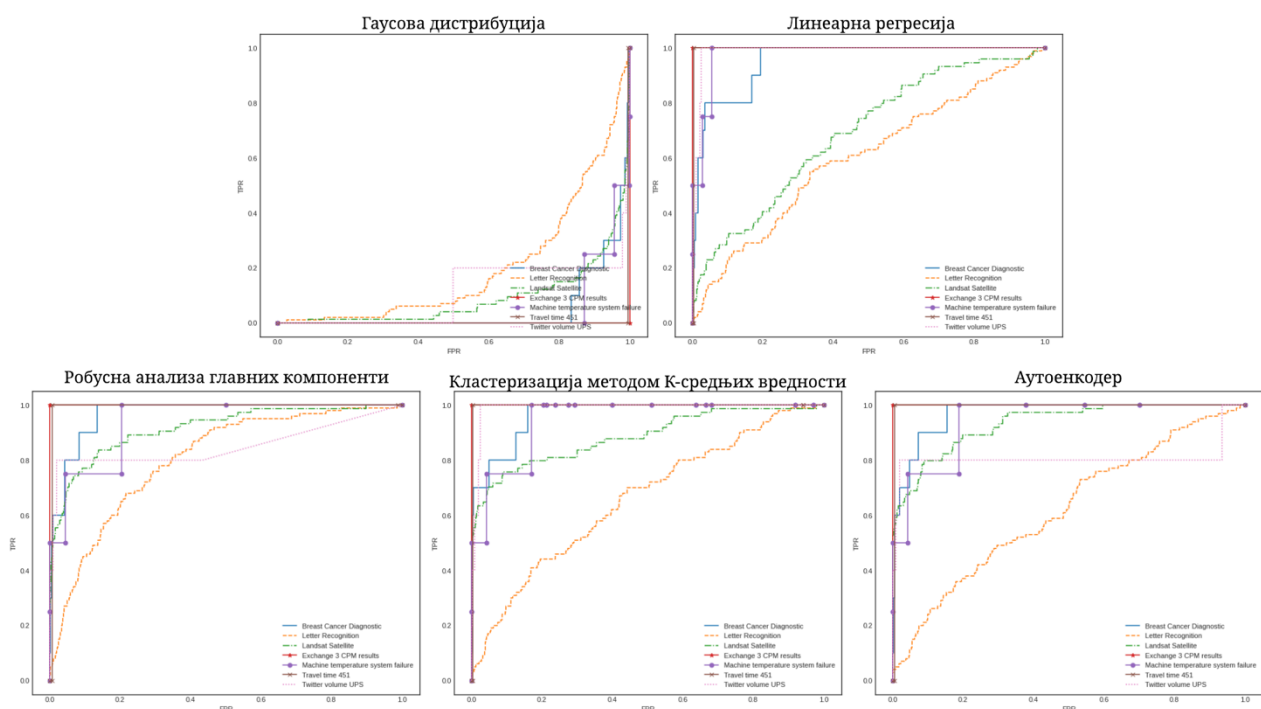
Слика 20: Анализа радне карактеристике пријемника за различите алгоритме и скупове података из различитих домена. Показано је да за различите домене података један алгоритам може да постигне другачије резултате за одређену оптимизациону метрику.
