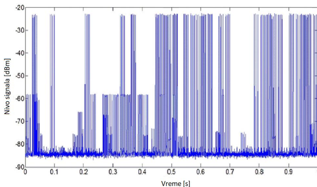
Slika 4.1 Signal prenosa podataka na radio interfejsu u uplinku preko GSM mreže, sekvenca trajanja 1 s
