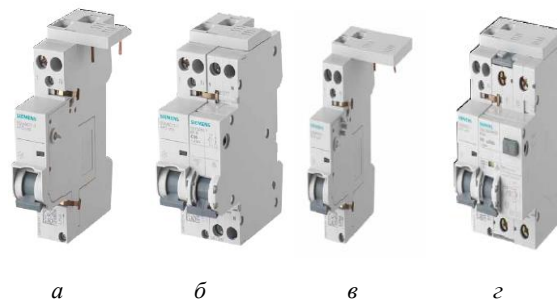
Слика 21. Заштитне 5SM6 AFDD компоненте а) и б) без и са аутоматским прекидачем, в) и г) без и са ЗУДС-ом
