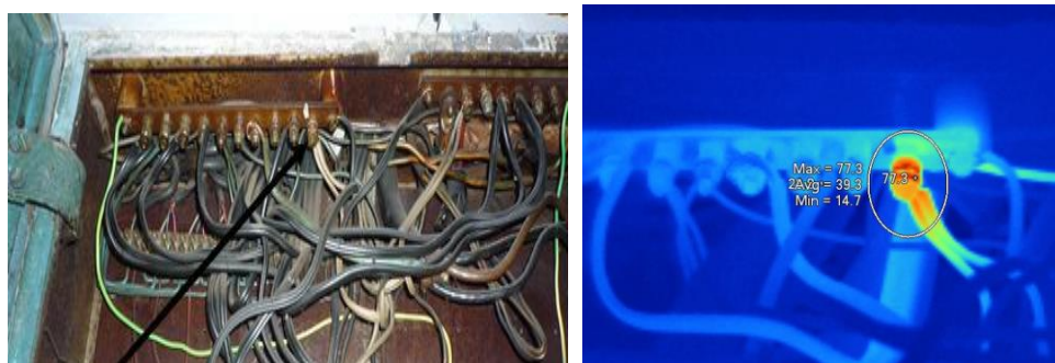
Слика 19. Пример термографијског снимка на коме се види „врела“ тачка на сабирници
