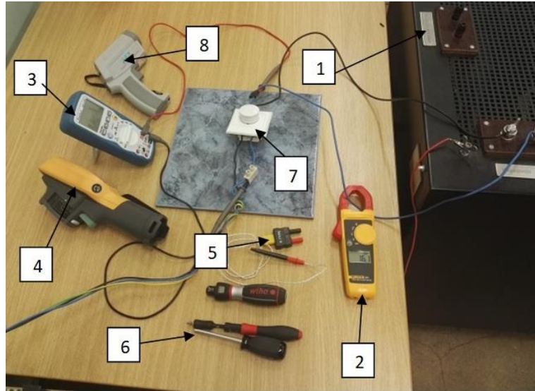
Слика 43. Експериментална поставка за анализу ефекта редукације момента затезања завртња на загревање електричних контаката у утикачима и утичницама (1. отпорничка кутија, 2. струјна клешта, 3. мултиметар (прецизан волтметар), 4. термовизијска камера, 5. термопар, 6. дигитални и механички „момент-шрафцигери“, 7. испитивана утичница или утикач, 8. ласерски мерач температуре)
