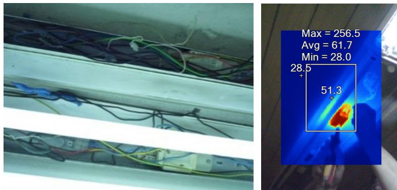
Слика 18. Прегревавање електромагнетске пригушнице у светиљци са флуо цевима
