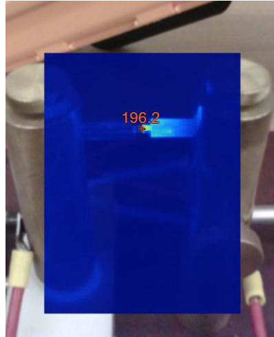
Слика 35. Пример термовизијске слике „вреле“ тачке за комбинацију електрода бакар–нерђајући челик
