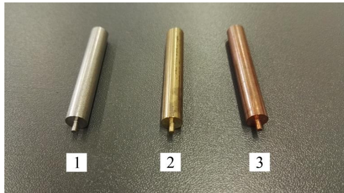
Слика 28. Испитне електроде по попречног пресека 1,5 mm 2 од нерђајућег челика (1), месинга (2) и бакара (3)
