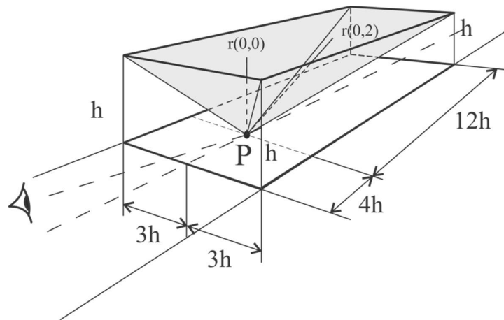
Слика 15. Просторни угао за израчунавање средњег коефицијента сјајности (h је висина оптичког центра светилке)
