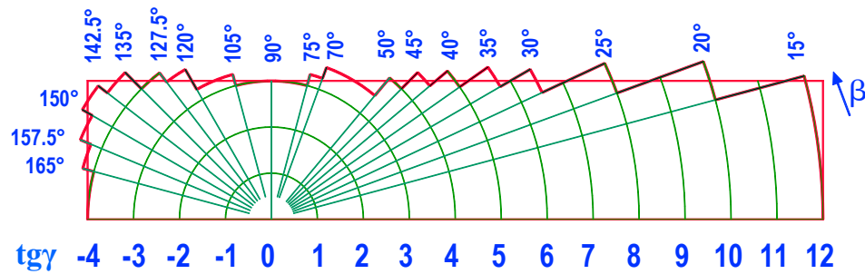
Слика 17. Границе интеграције по променљивим \text{tg}\gamma и \beta , приказане у равни коловоза
