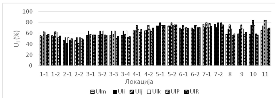
Слика 43. Измерене ( U_{lm} ) и израчунате вредности ( U_{li} , U_{lj} , U_{lk} , U_{lP} and U_{lR} ) подужне равномерности сјајности
