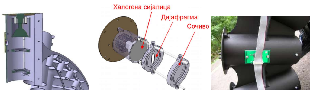
Слика 34. Извор светлости са припадајућим оптичким системом (изглед, подушни пресек и спољни изглед са приказаном фотоћелијом за аутокалибрацију)
