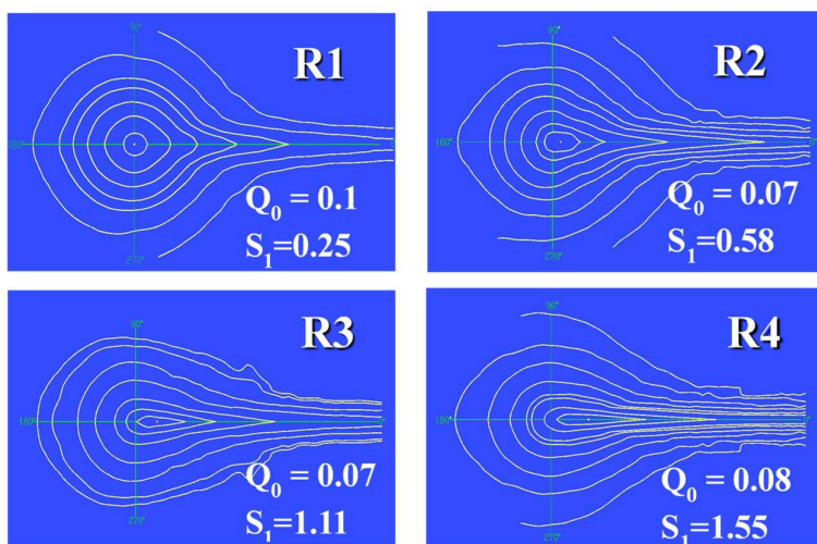
Слика 22 Изо-г дијаграми стандардних рефлексивних класа коловоза
