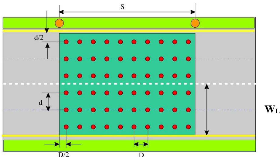
Слика 4. Распоред тачака вредновања при прорачуну сјајности
