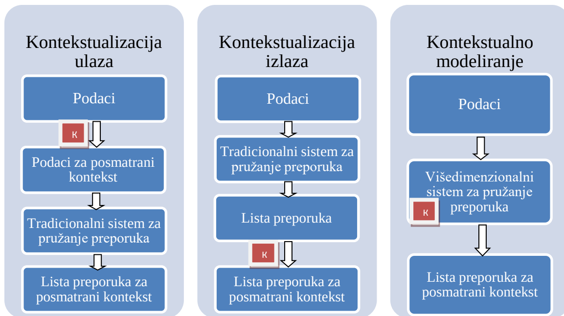
Slika 4.2: Tri načina korišćenja kontekstualnih informacija u sistemu [13].
