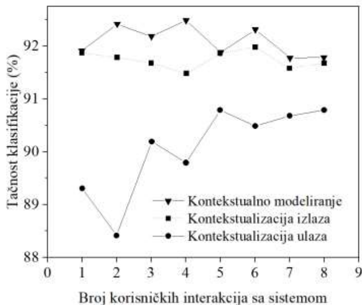
Slika 7.5: Poređenje sistema koji na različite načine koriste kontekstualne informacije.
