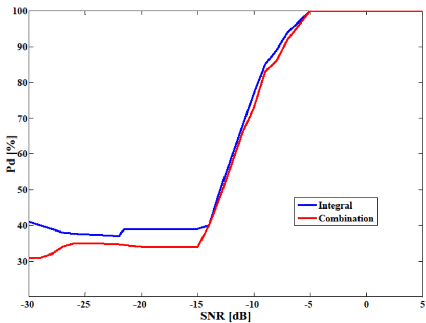
Слика 33: Перформансе алгоритама за анализу спектра у каналу са AWGN и за 16-QAM модулисане PU сигнале.
