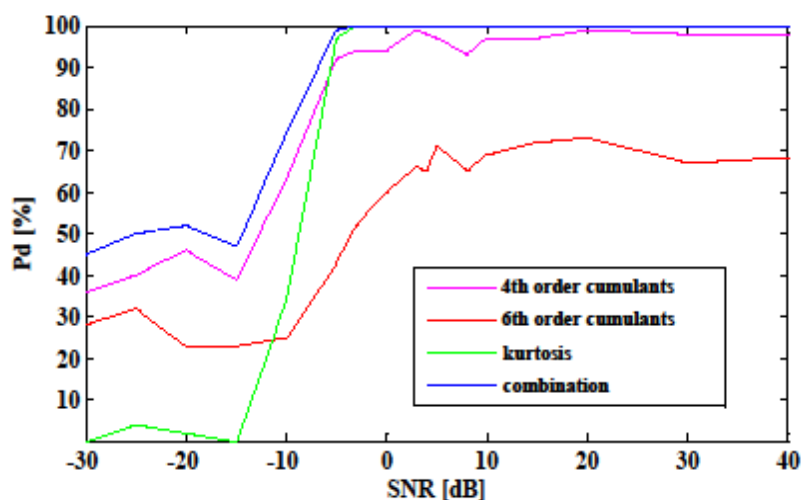
Слика 29: Перформансе различитих алгоритама за анализу спектра у каналу са AWGN и вишеструком пропагацијом непознатог импулсног одзива и за 64-QAM модулисане PU сигнале.
