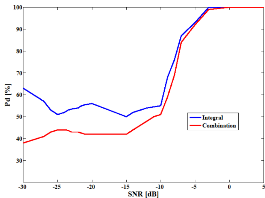
Слика 35: Перформансе алгоритама за анализу спектра у каналу са вишеструком пропагацијом непознатог импулног одзива и AWGN, и за QPSK модулисане PU сигнале.
