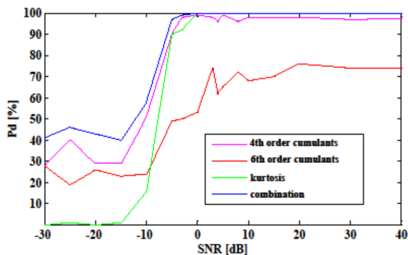
Слика 28: Перформансе различитих алгоритама за анализу спектра у реалном каналу са AWGN и вишеструком пропагацијом непознатог импулсног одзива и за 16-QAM модулисане PU сигнале.
