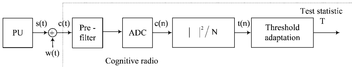
Слика 17: Блок шема модела детектора енергије.
