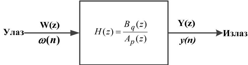
Слика 19: Релације између улазних и излазних сигнала AR процеса.
