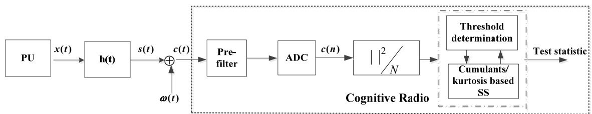
Слика 30: Модел интегралног алгорита за анализу спектра у когнитивном радију на бази детектора енергије и статистичке обраде примљеног сигнала.
