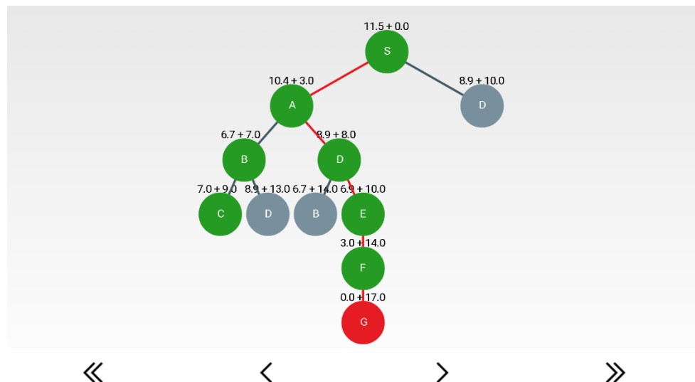
Слика 42 - Стабло претраживања за симулацију алгорита A^*
