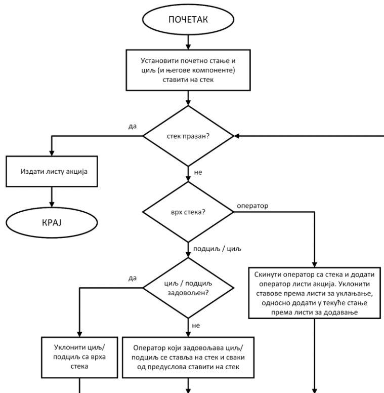
Слика 6 – Дијаграм извршавања алгорита STRIPS
