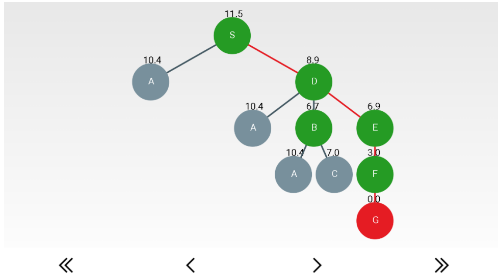
Слика 41 - Стабло претраживања за симулацију алгорита прво најбољи
