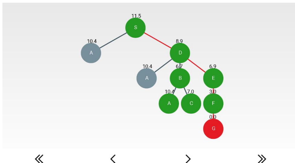
Слика 40 - Стабло претраживања за симулацију алгорита планинарења
