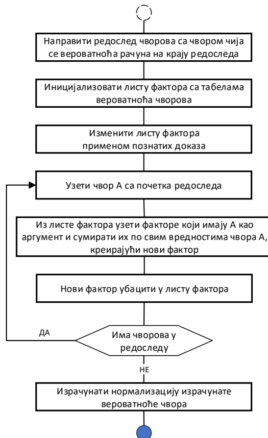
Слика 4 - Дијаграм алгоритма елиминације чворова
