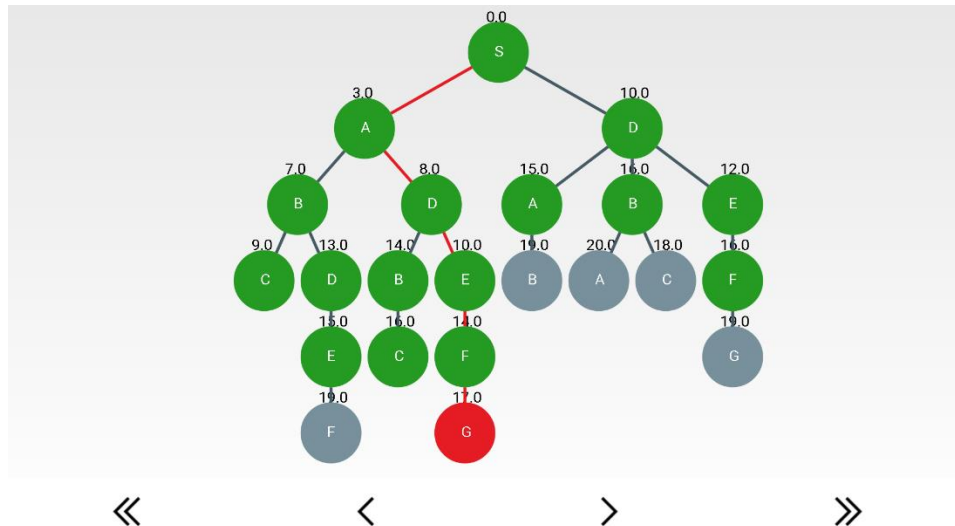
Слика 39 – Стабло претраживања за симулацију алгорита гранања и ограничавања
