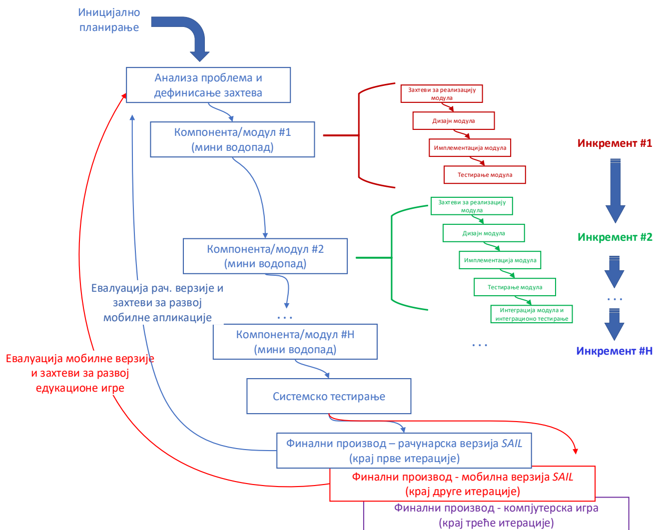
Слика 9 - Модел развоја софтверског система SAIL
