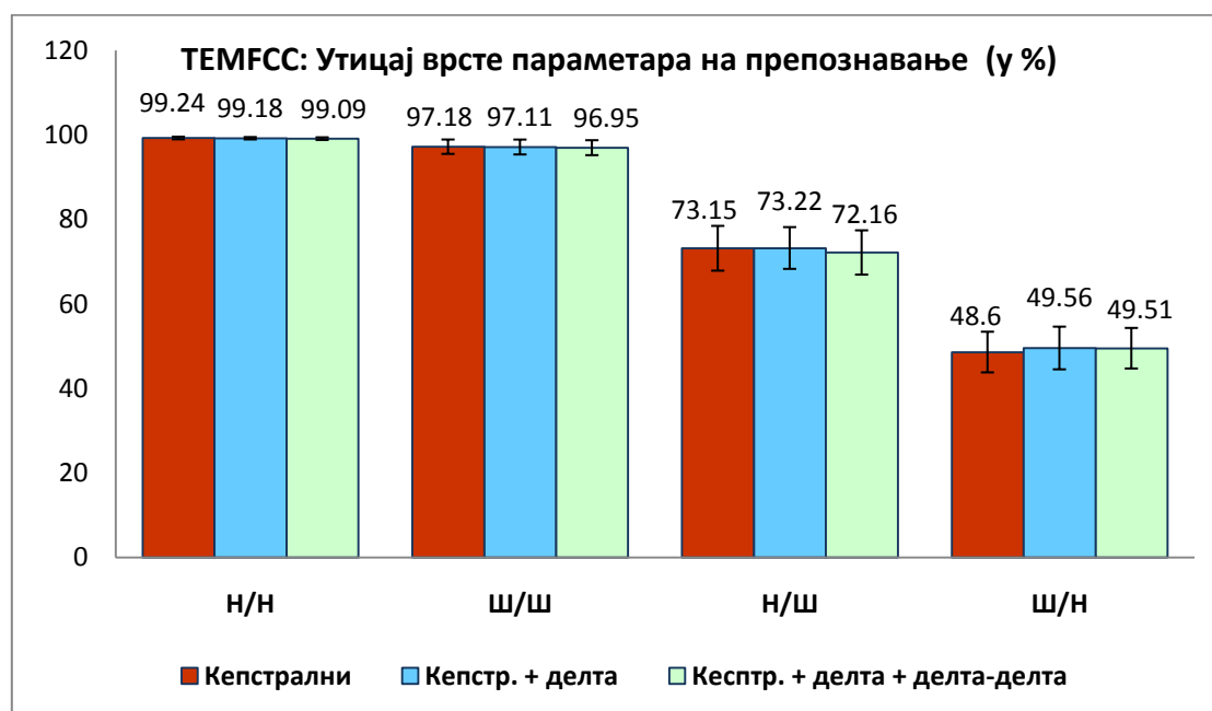
Слика 6.18 Утицај врсте параметара на препознавање за TEMFCC обележје.
