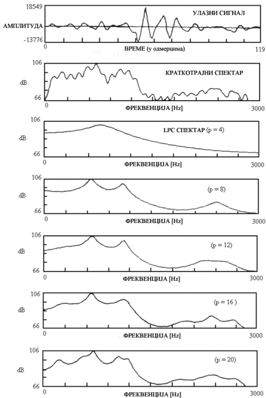
Слика 3.4 Зависност LPC спектра од реда аутокорејације p [Rabiner, Juang, 1993].
