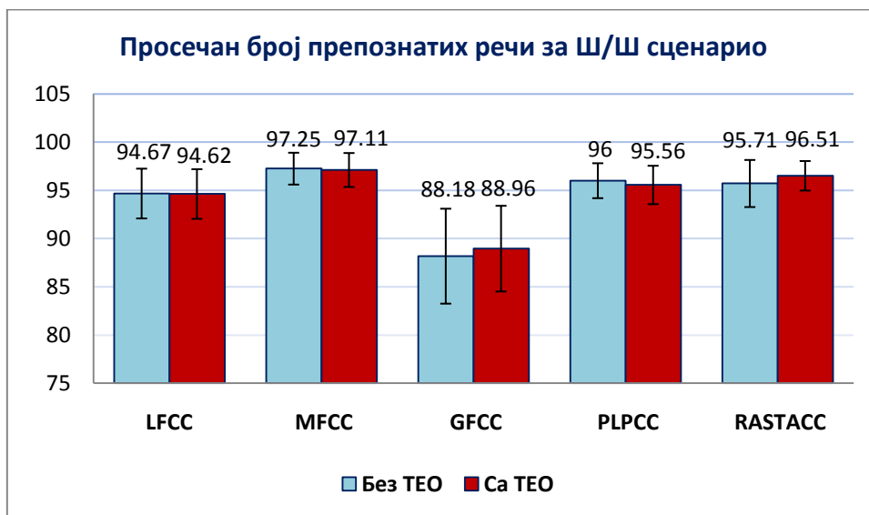
Слика 6.40 Просечан број препознатих речи за Ш/Ш сценарио без и са ТЕ оператором.
