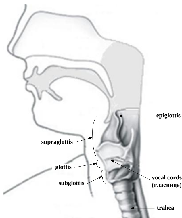
Слика 2.11 Глотални делови који утичу на шапат.
