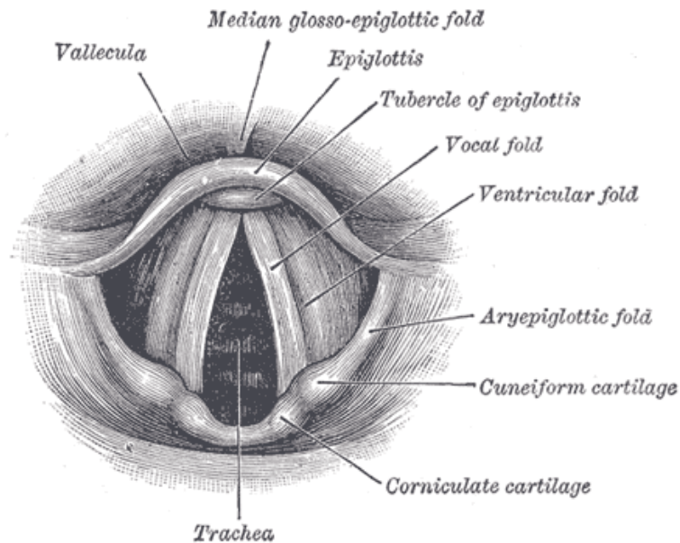
Слика 2.9 Глотис-детаљно [Wikipedia].
