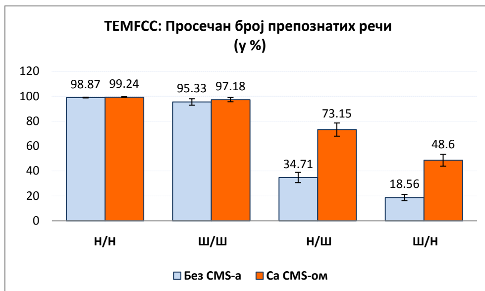
Слика 6.17 Резултати препознавања за TEMFCC обележје без и са CMS-ом.
